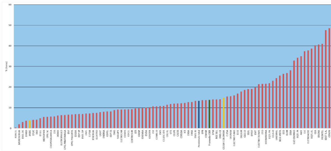
Gráfico 5.1: Tiempo total de interrupción por cliente (Tc horas) Total de incidencias
